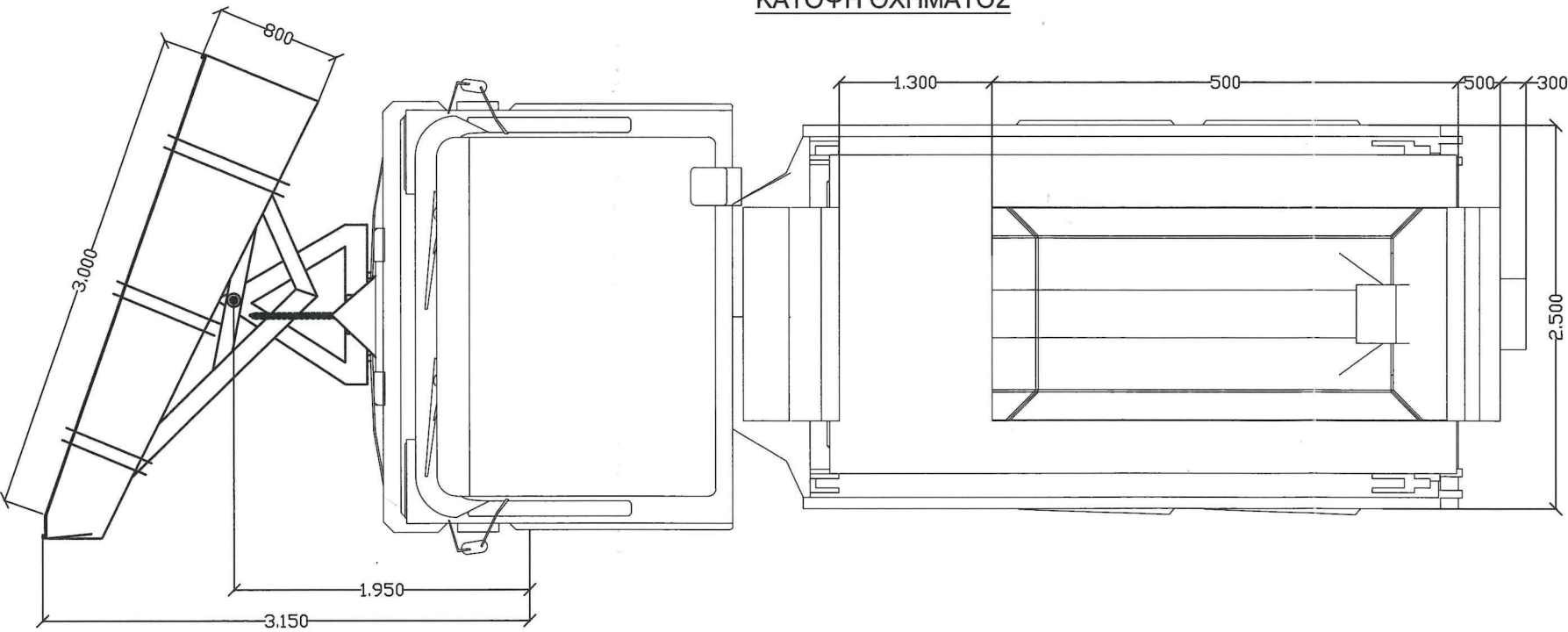
ΚΑΤΟΨΗ ΟΧΗΜΑΤΟΣ
