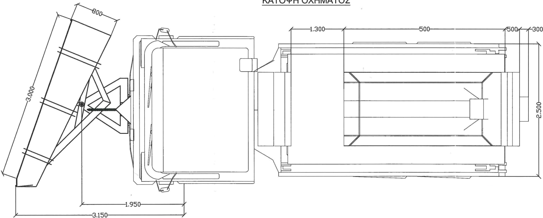
ΚΑΤΟΨΗ ΟΧΗΜΑΤΟΣ
