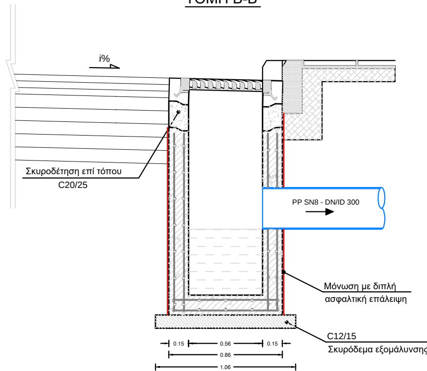
ΤΟΜΗ Β-Β'
