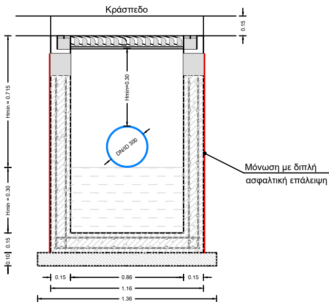
ΤΟΜΗ Α-Α'
