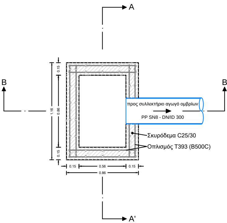
ΚΑΤΟΨΗ
