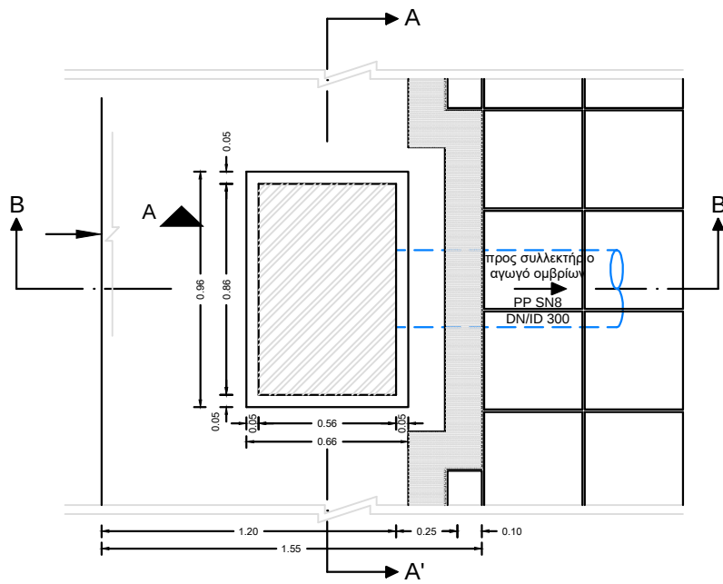
ΑΝΟΨΗ
