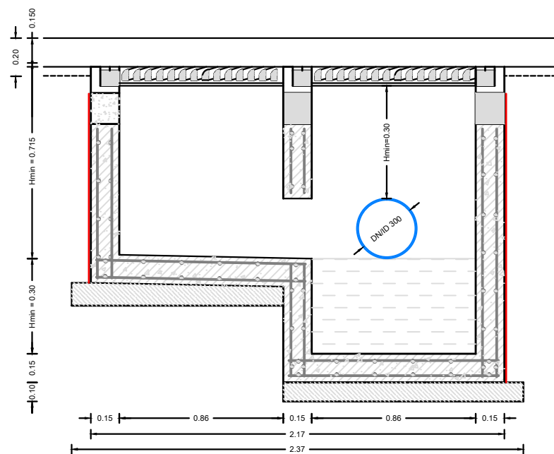
ΤΟΜΗ Α-Α' (δίδυμο φρεάτιο)
