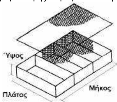
Σχήμα 2: Στρώμη τύπου RENO με διαφράγματα
