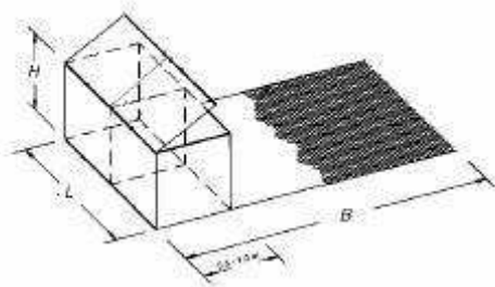
Σχήμα 4: Συρματοκιβώτια με προέκταση συρματοπλέγματος τύπου TERRAMESH.
