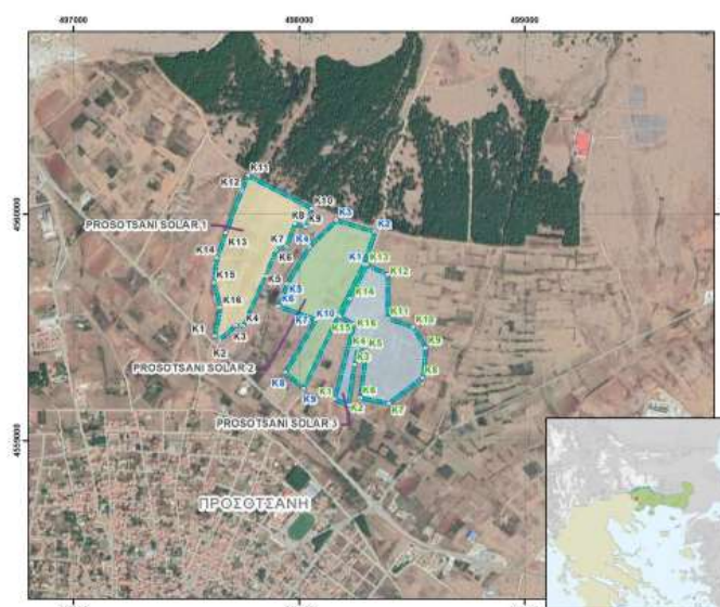
Σχήμα 1.3.: Γενική απεικόνιση των γεωτεμαχίων ανάπτυξης των Φ/Β Σταθμών.
